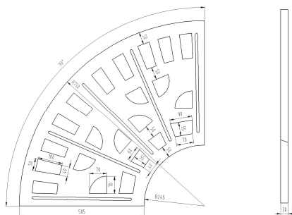
Vegetační mříž kruhová D150
