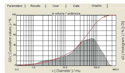
Granulometrie - záznam
